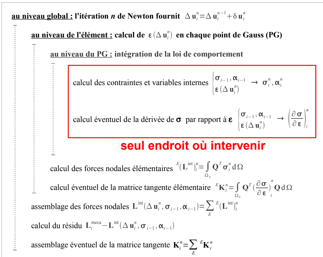
FIGURE 3 : Place de la loi de comportement dans le schéma itératif de recherche de l'équilibre.
