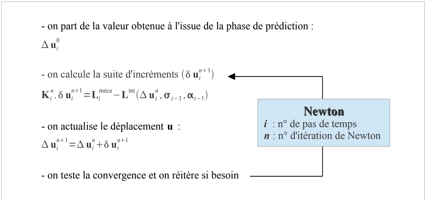
FIGURE 2 : Schéma général de résolution d'un problème non linéaire en mécanique des structures par la méthode de Newton-Raphson.
