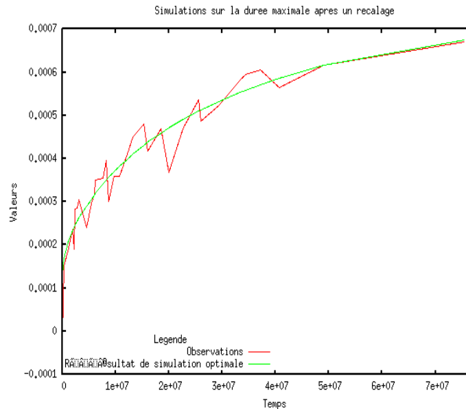
FIGURE 12 : courbe expérimentale et recalée
